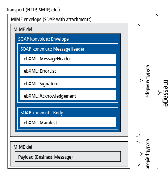
Figuren viser hvordan en ebXML-melding pakkes.
